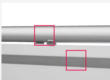
Plis en haut pour renfort et liaison avec la main courante Fixations par rivet pop pour la main courante intégrés dans la tôle
