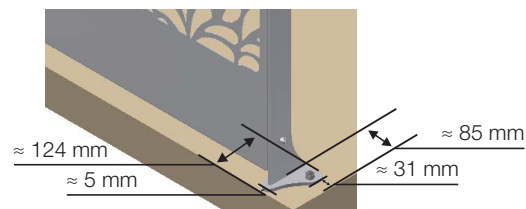
Décalage par rapport au périmètre de la zone à protéger
